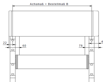
Draufsicht einteilig (Getriebe)
