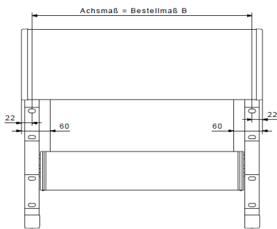
Draufsicht einteilig (Motor)
