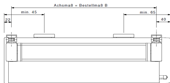
Vorderansicht einteilig (Getriebe)
