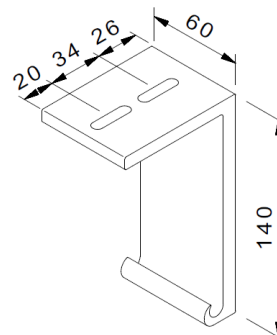
Deckenkonsole
