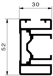
Führungsschiene
