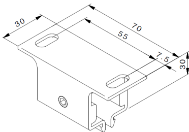
Führungsschienenhalter
