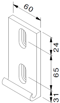
Wandkonsole
