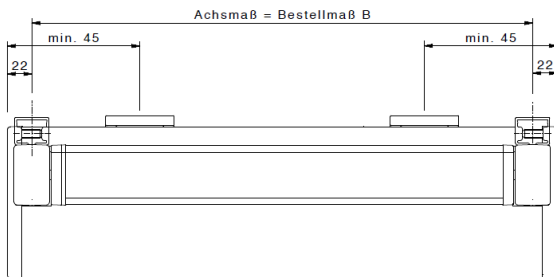
Vorderansicht einteilig (Motor)
