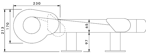
Vorderansicht einteilig
