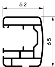
Führungsschiene
