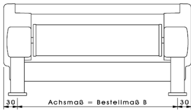
Vorderansicht einteilig
