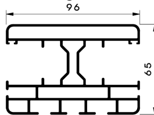
Mittelführungsschiene
