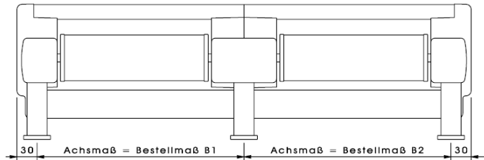
Vorderansicht zweiteilig
